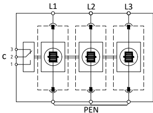
Принципиальная схема
